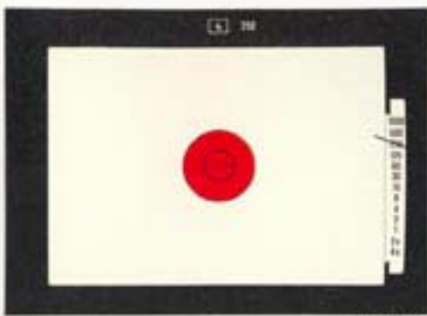
Ci-dessus: Champ de la mesure sélective En haut à gauche: Champ de la mesure intégrale Ci-contre: Répartition de la sensibilité dans la mesure intégrale LEITZ.
