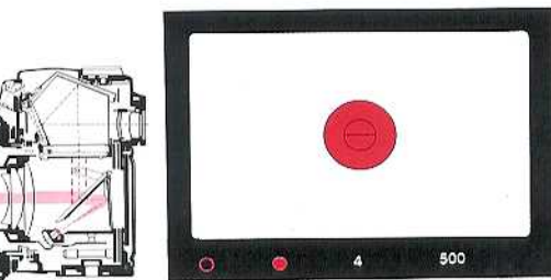
Représentation schématique de la mesure sélective LEICA
